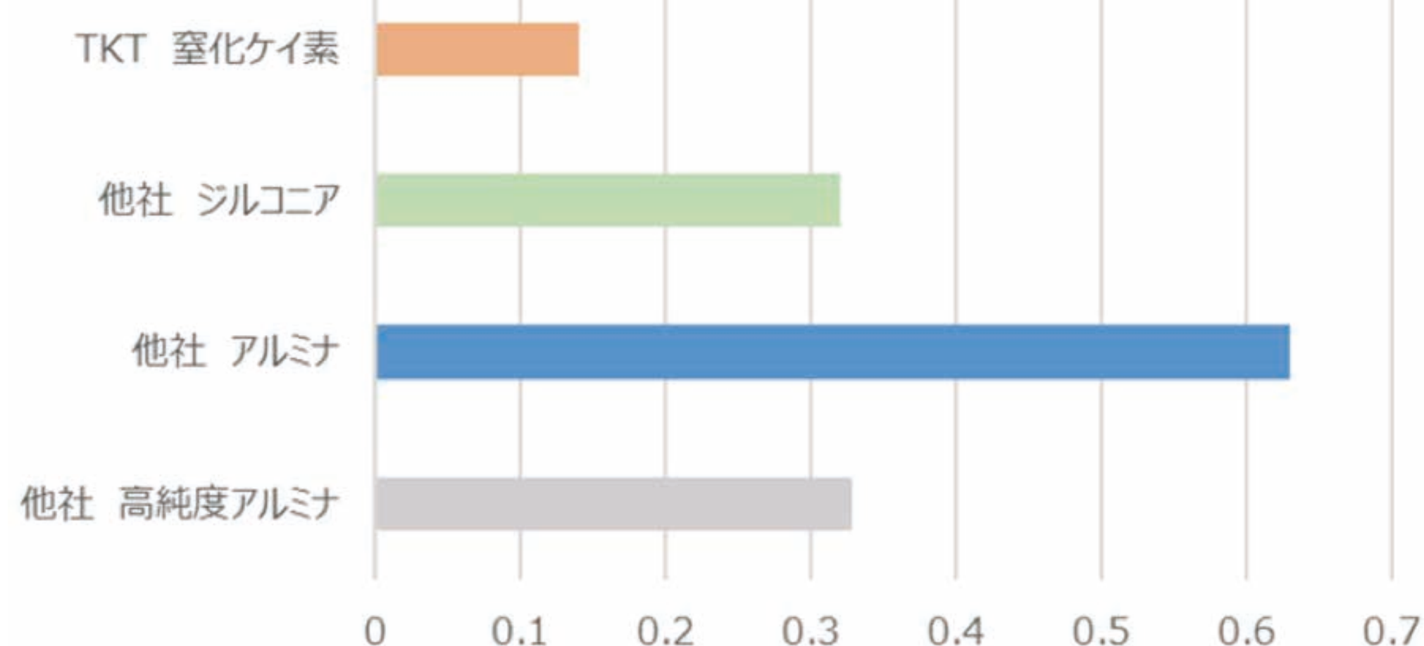
他材質との摩耗減少率比較結果
