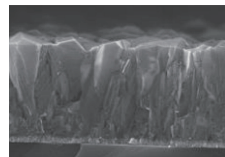
断面写真
